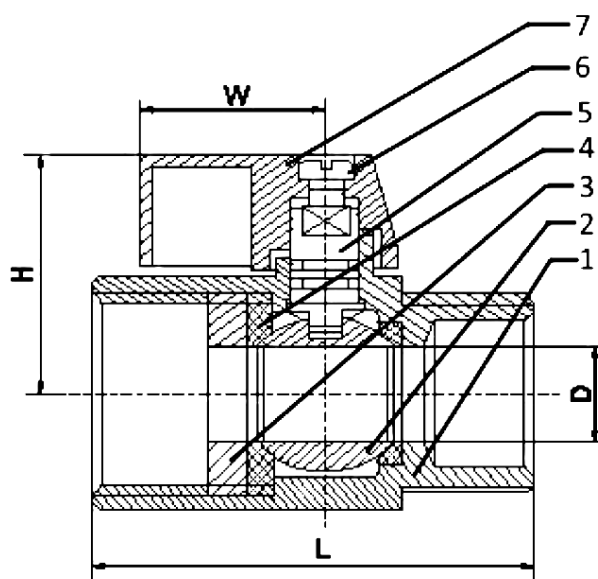
SS316 M x F Mini Ball Valve Drawing
